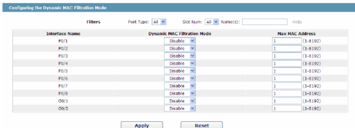
Рисунок 14 Настройки режима динамической MAC фильтрации
