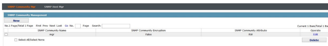
Рисунок 2: Управление SNMP
